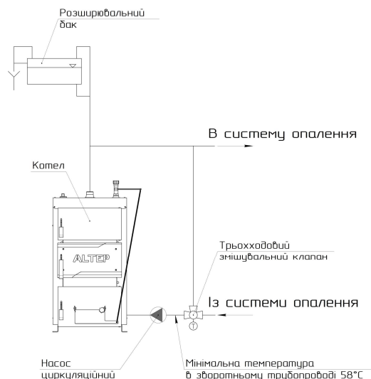
Рисунок 4 – Схеми підключення котла до системи опалення
