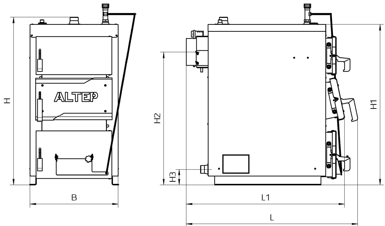
Рисунок 1 – Габаритне креслення котла Altep-Compact
